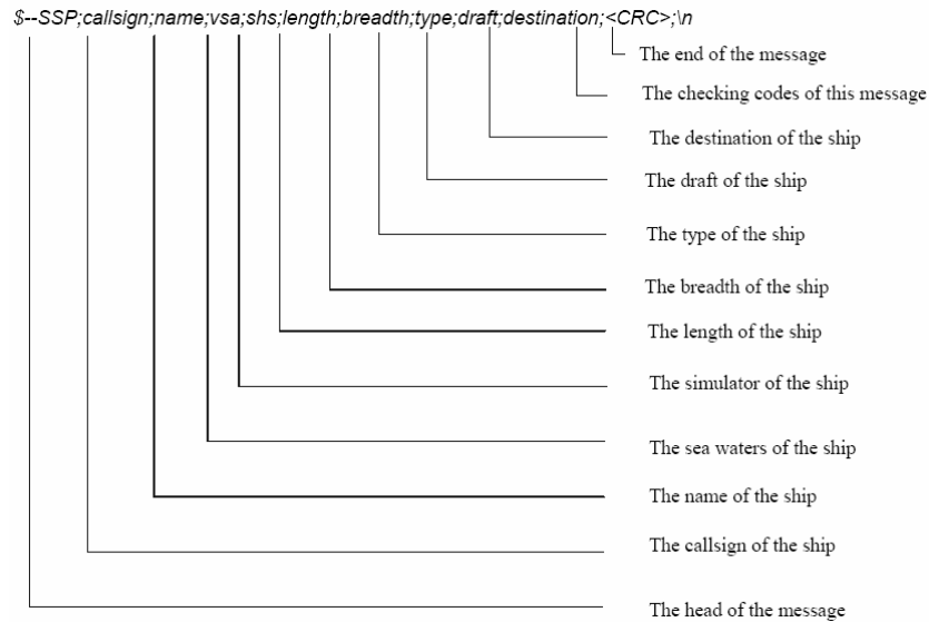
Fig. 6 The format of message SSP
